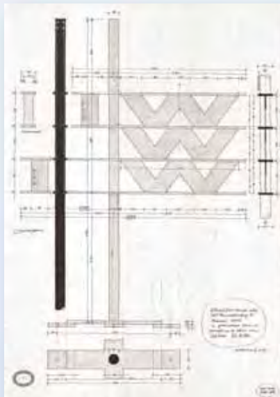
Het definitieve ontwerp voor een windwijzer op het trappenhuis aan de binnenhof tussen de oude abdij van Vaals en de nieuwe bibliotheek. Een ontwerp van dom Hans van der Laan uit 1986. De letters kunnen – naar gelang de windrichting – worden gelezen als: Ik Waai Waar Ik Wil, of Waar Ik Wil Waai Ik (Johannes 3, vers 7-9). Zie ook pagina 187.
